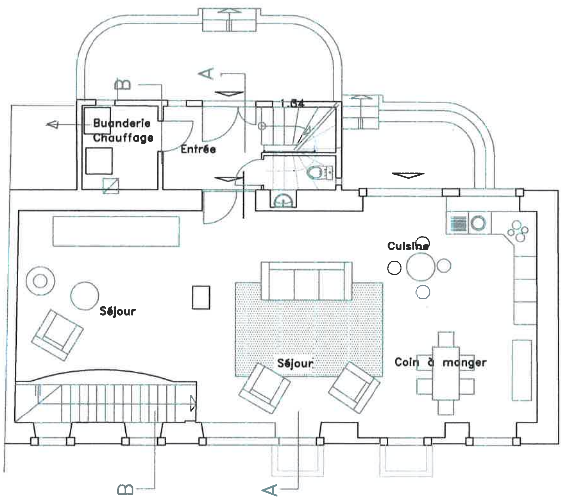
Rez-de-chaussée
