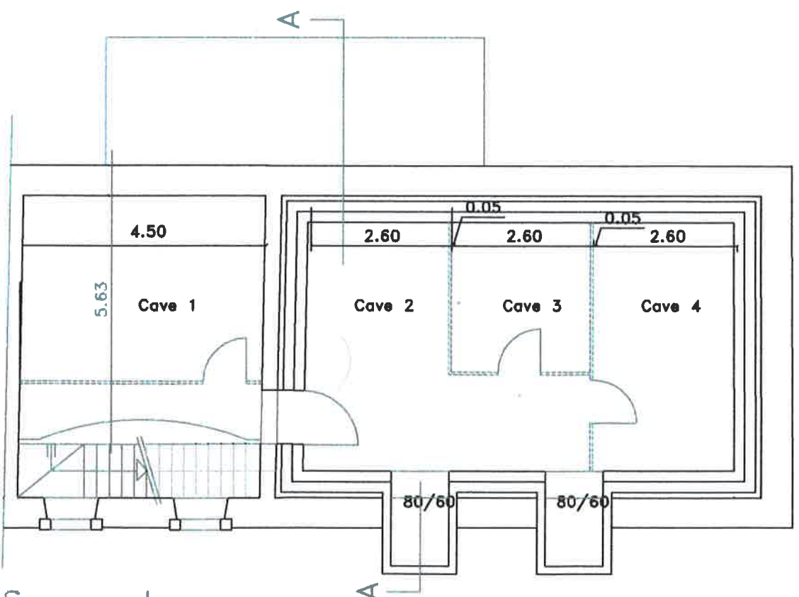
Sous-sol
